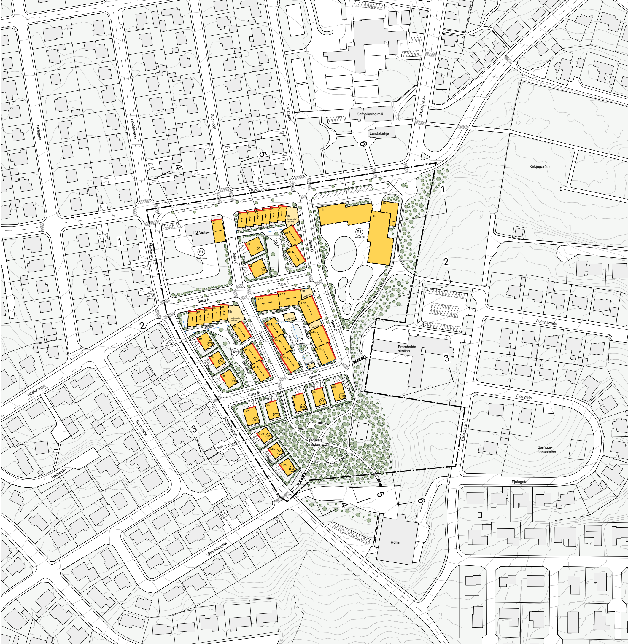
Deiliskipulagsuppráttur // Mkv. 1:2000
